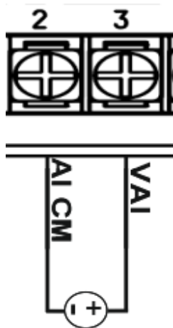
اتصال سیگنال ولتاژ
