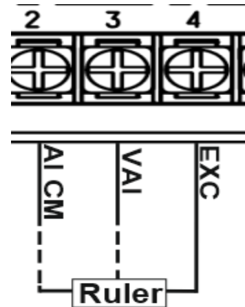
اتصال خطکش مقاومتی
